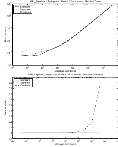
Fig. 6. MPI_Allgather
