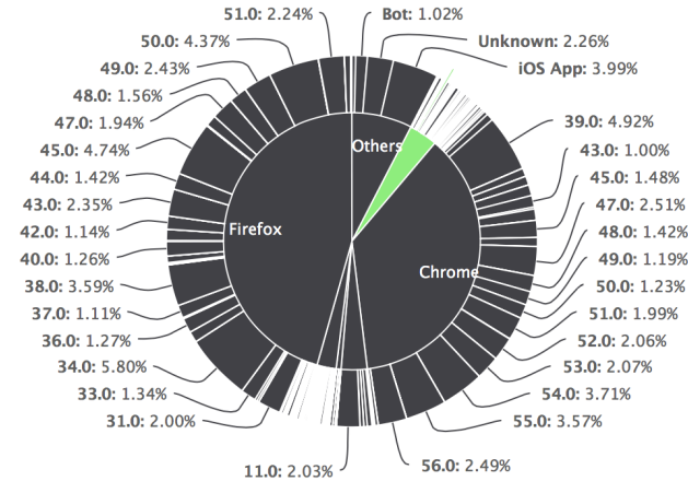
Browser
