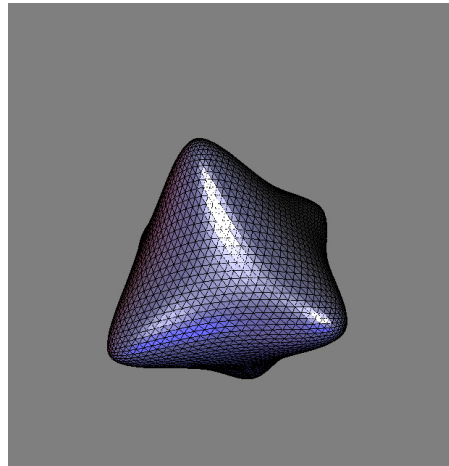
subdivision level 4
