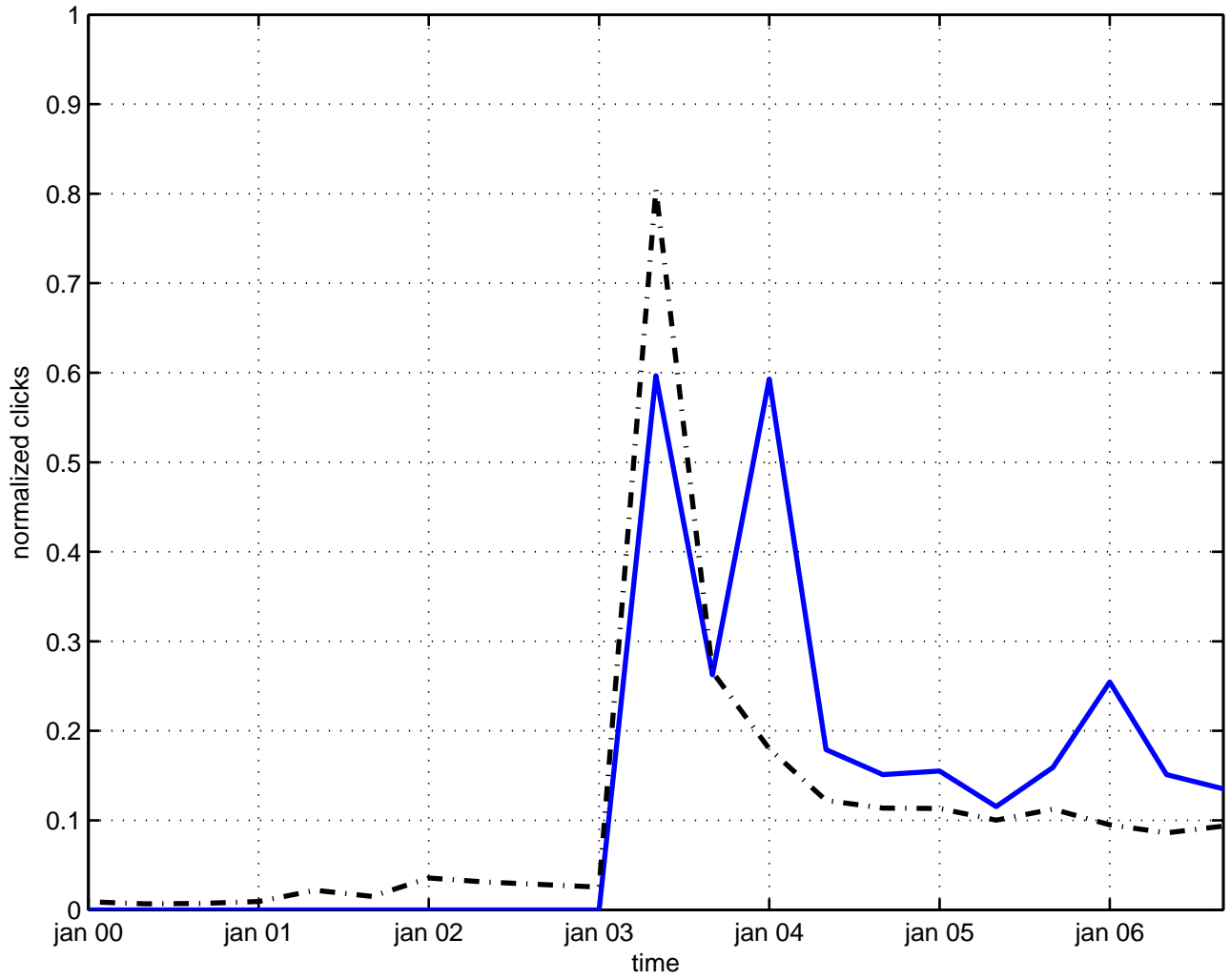
zero mode vortex
