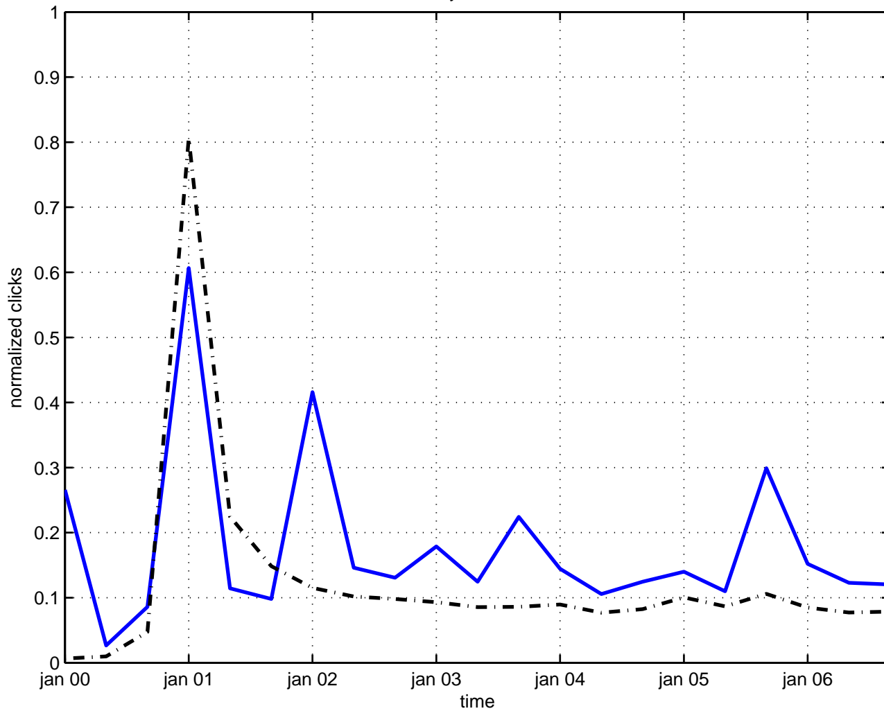
weyl fermion
