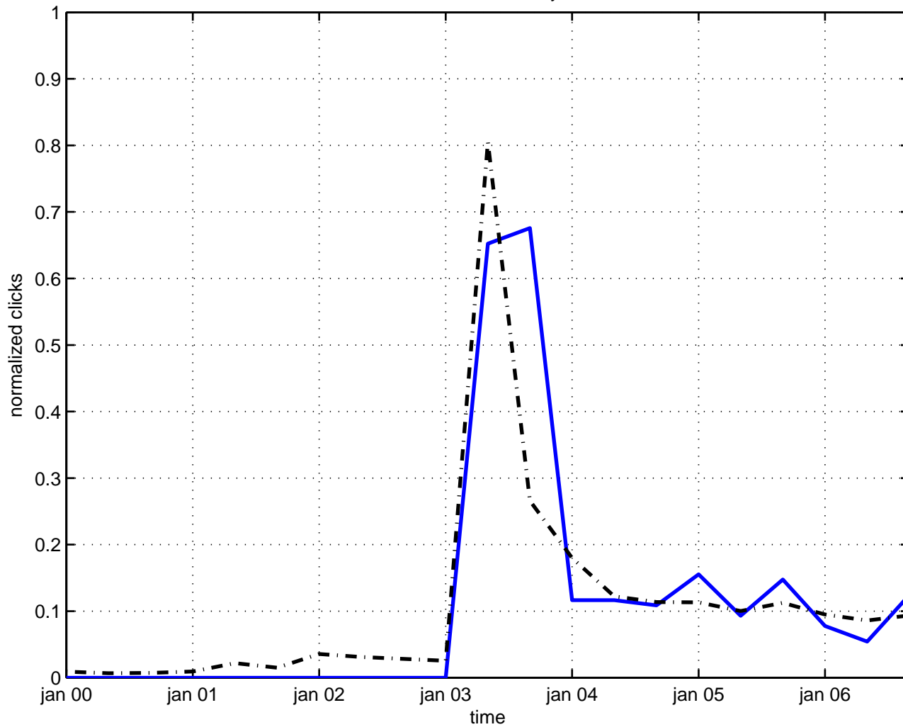
virasoro anomaly
