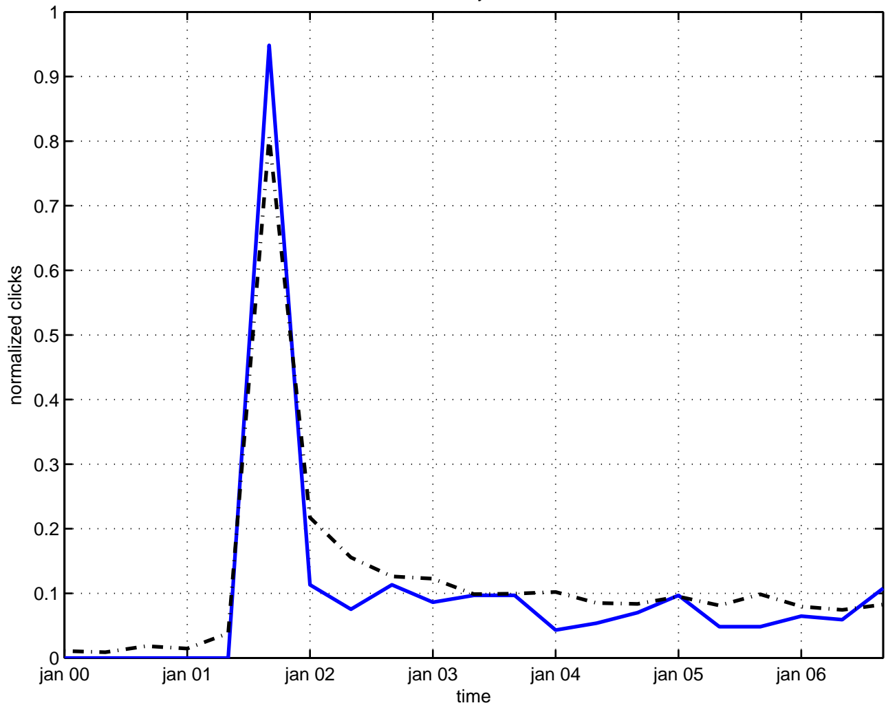
universality fermion
