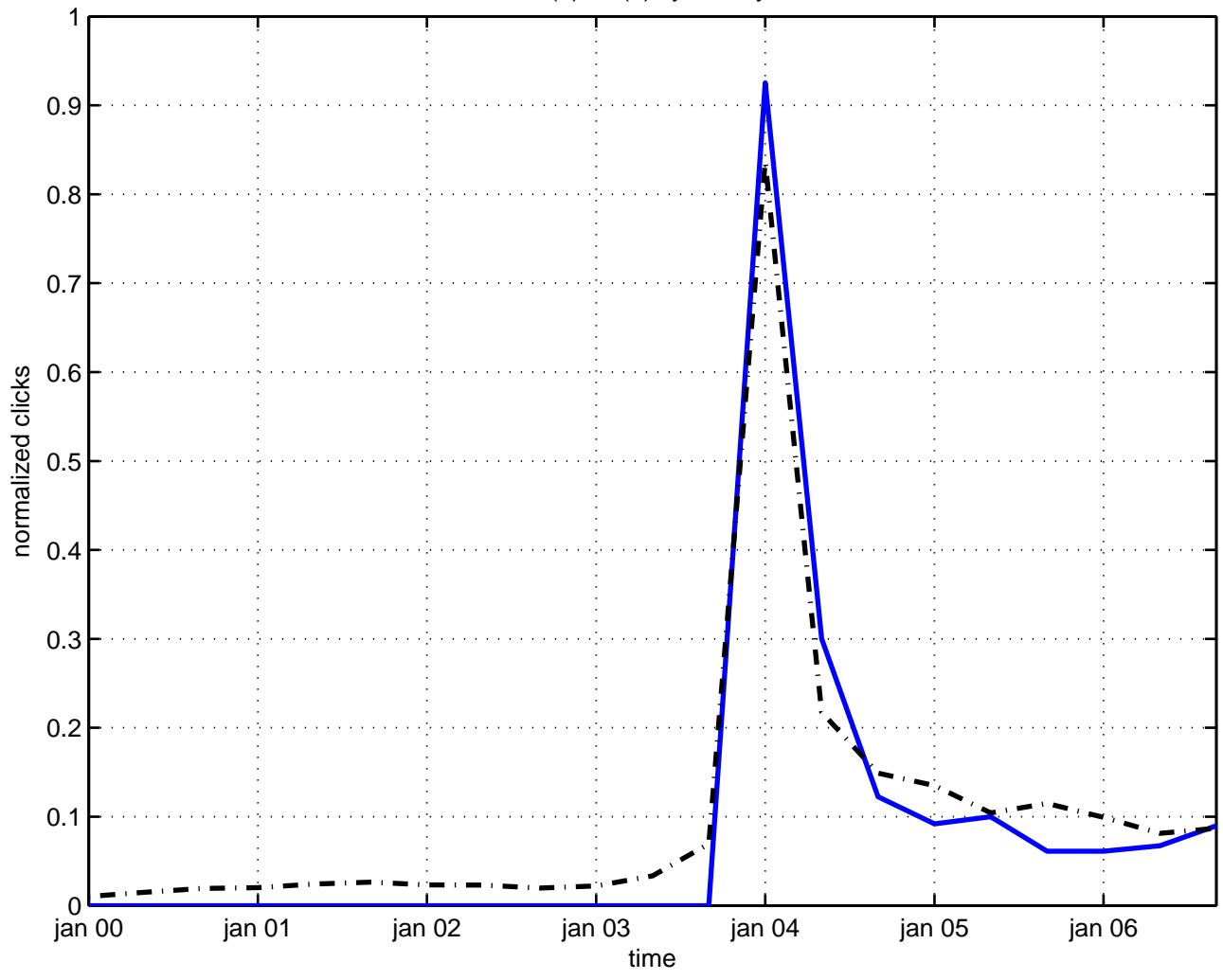
u(n) x u(n) symmetry
