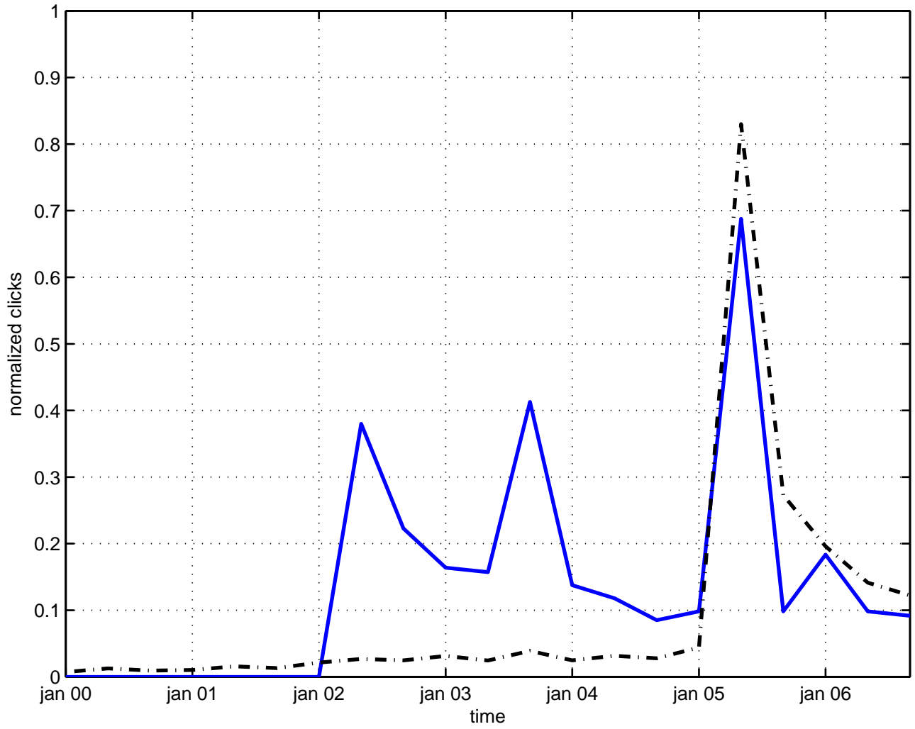
u(n) invariance
