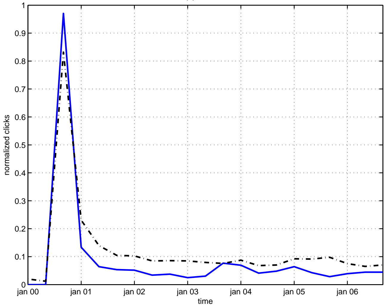
u(n) instanton
