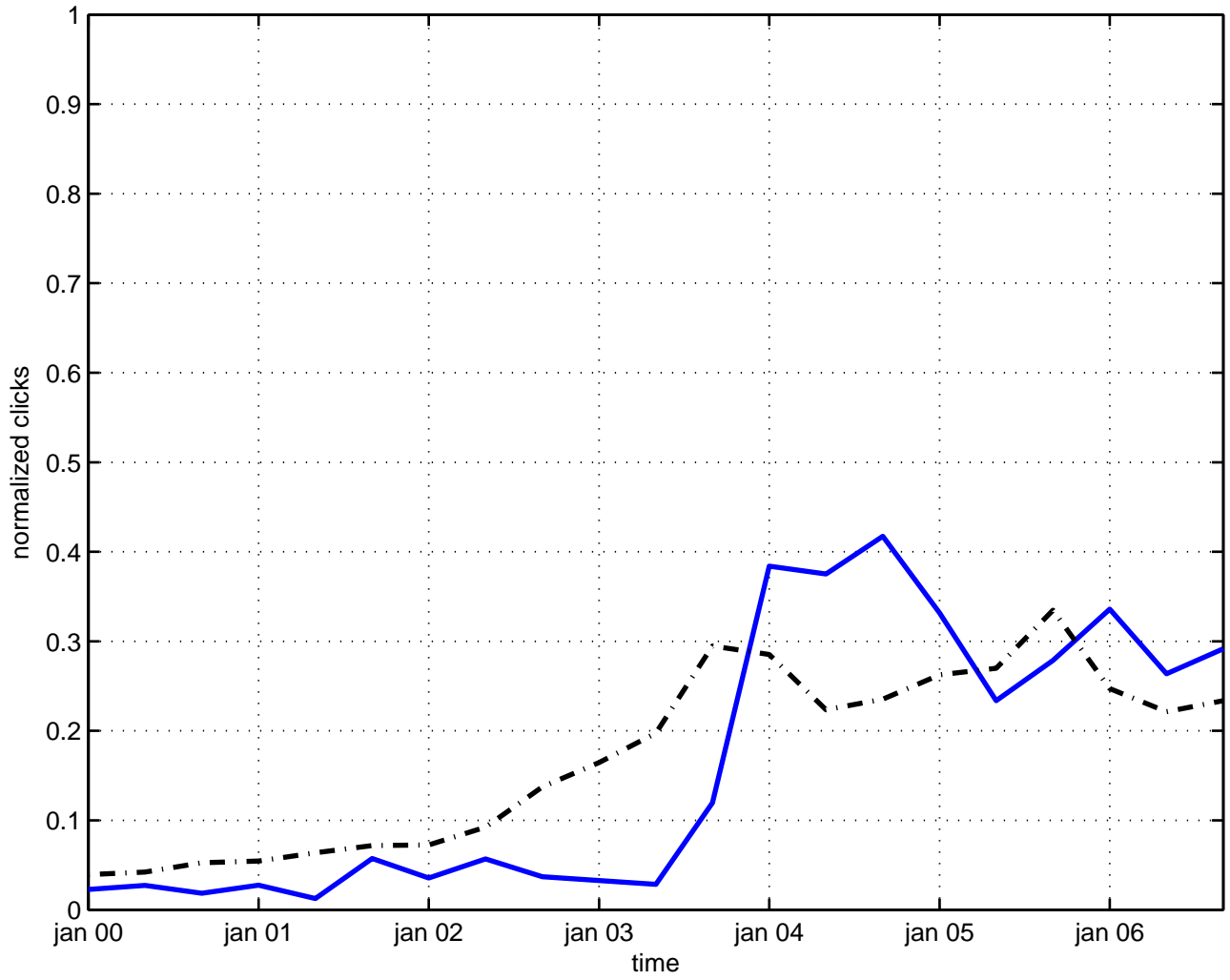
twistor
