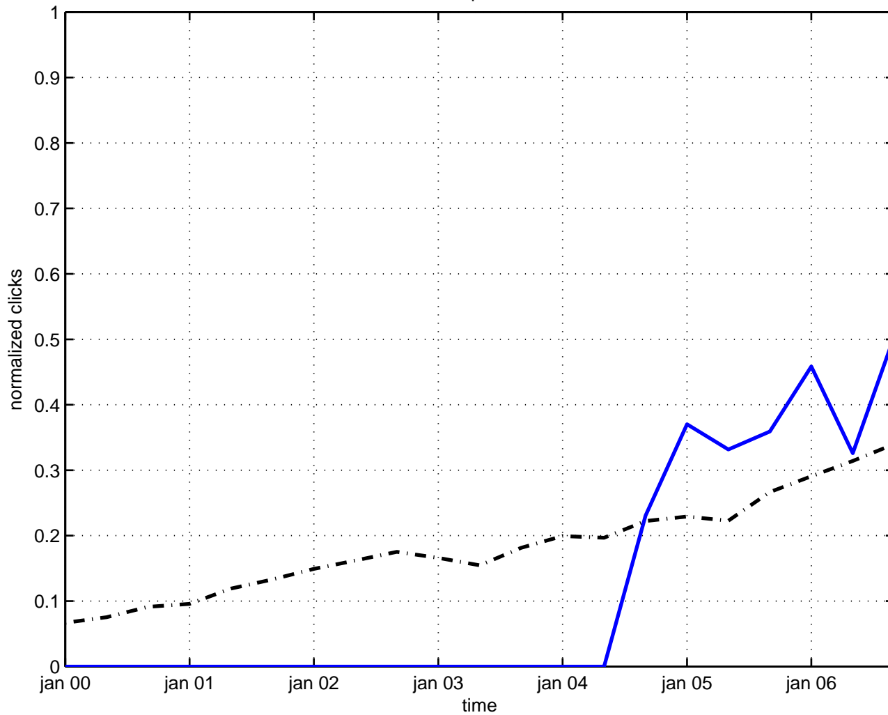
torus compactification
