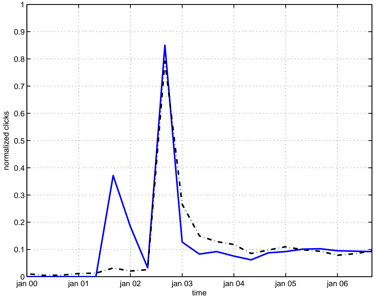
theta parameter quantum chromodynamics
