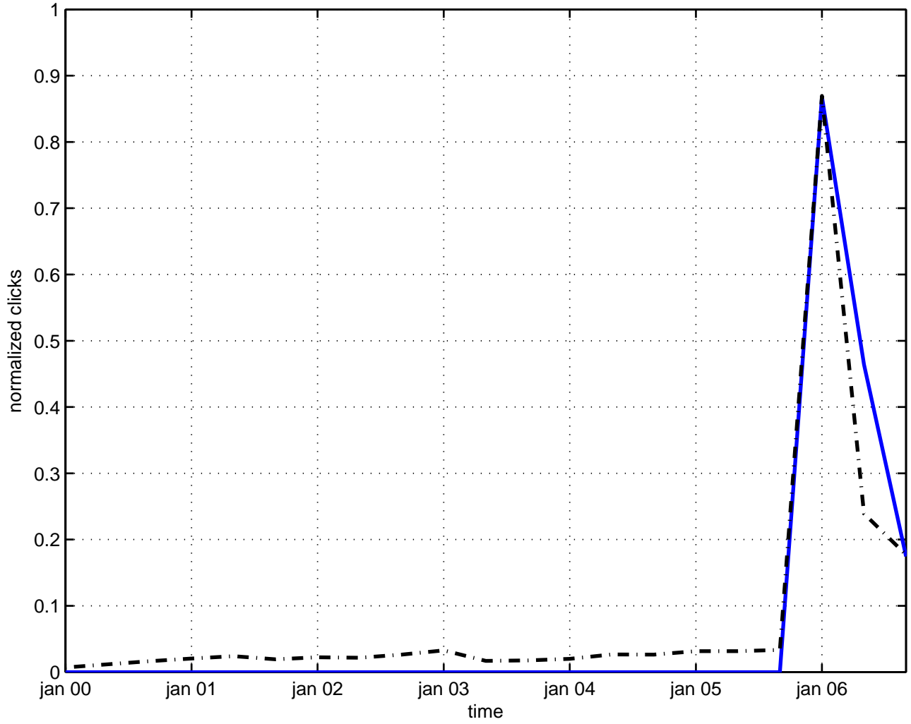
t(6)/z(4) orientifold
