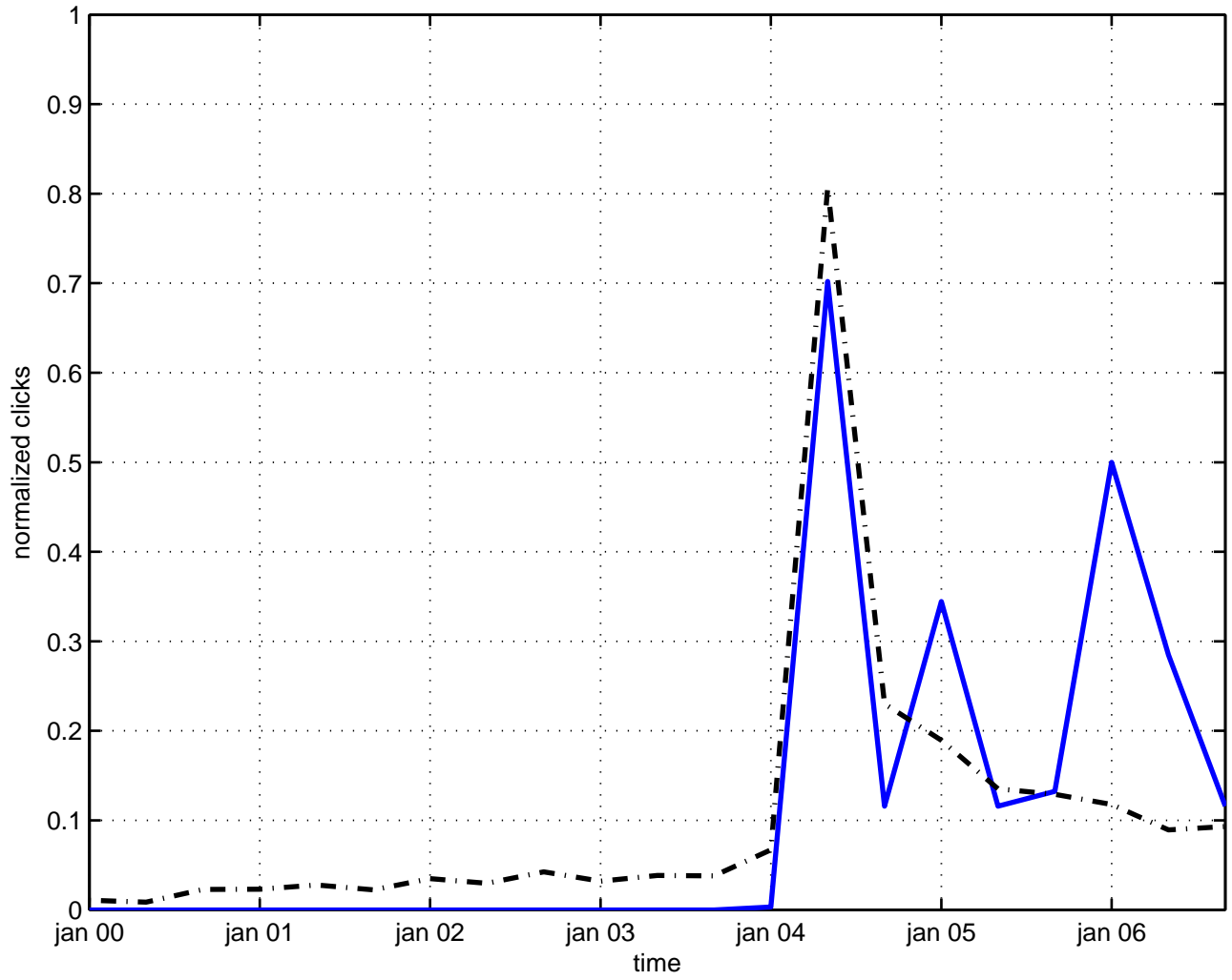
superradiance
