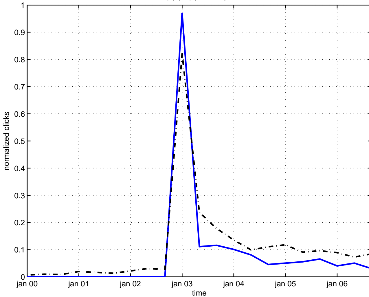
su(n|1)/u(n) coset space
