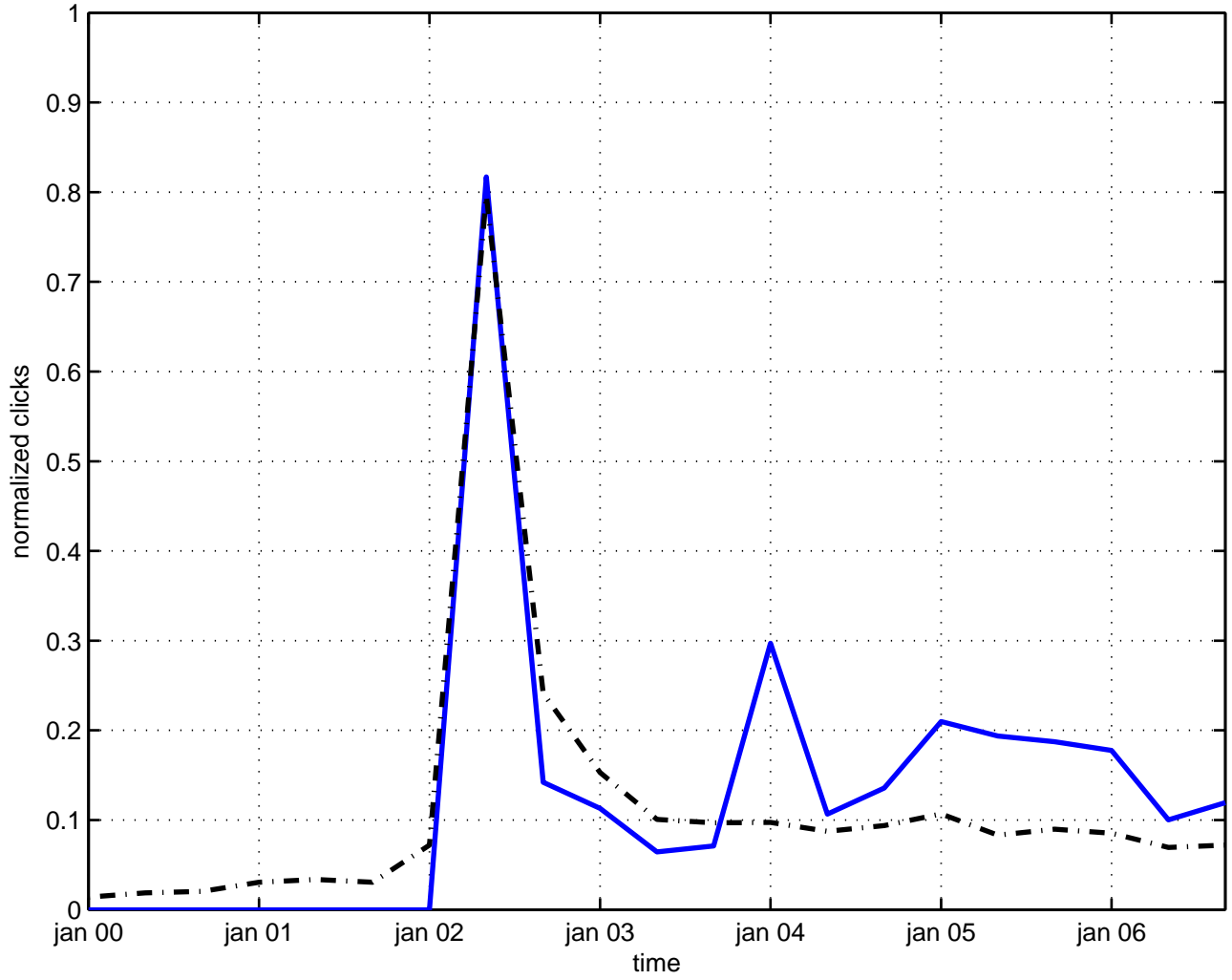
string boson
