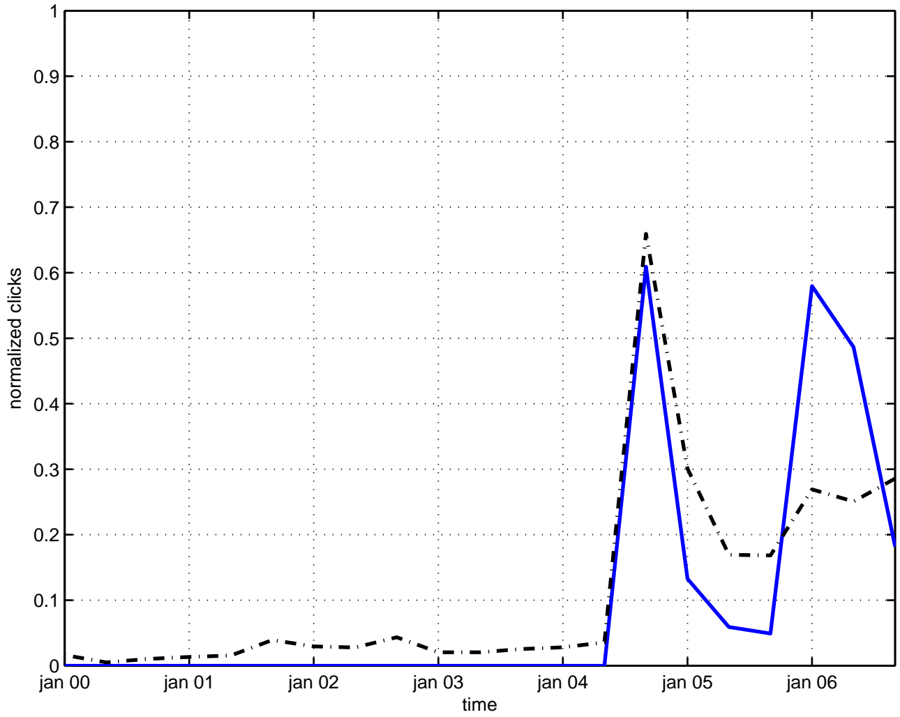
star boson
