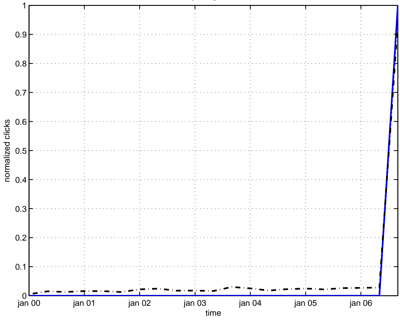
spin skyrmion
