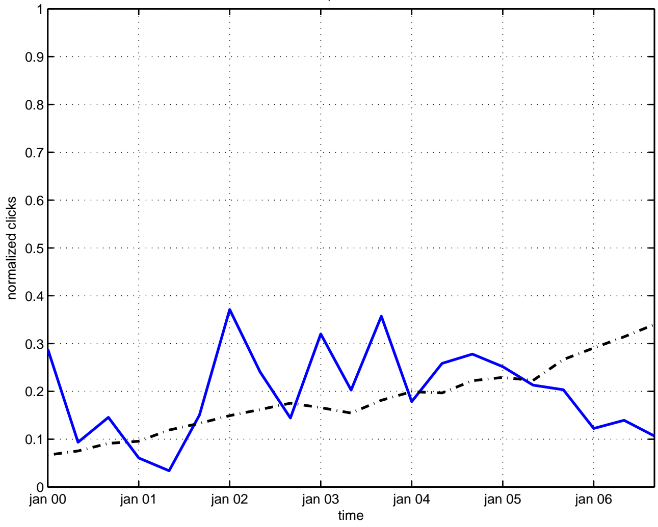
sphaleron
