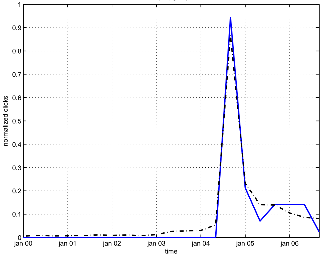
sl(3,c) group
