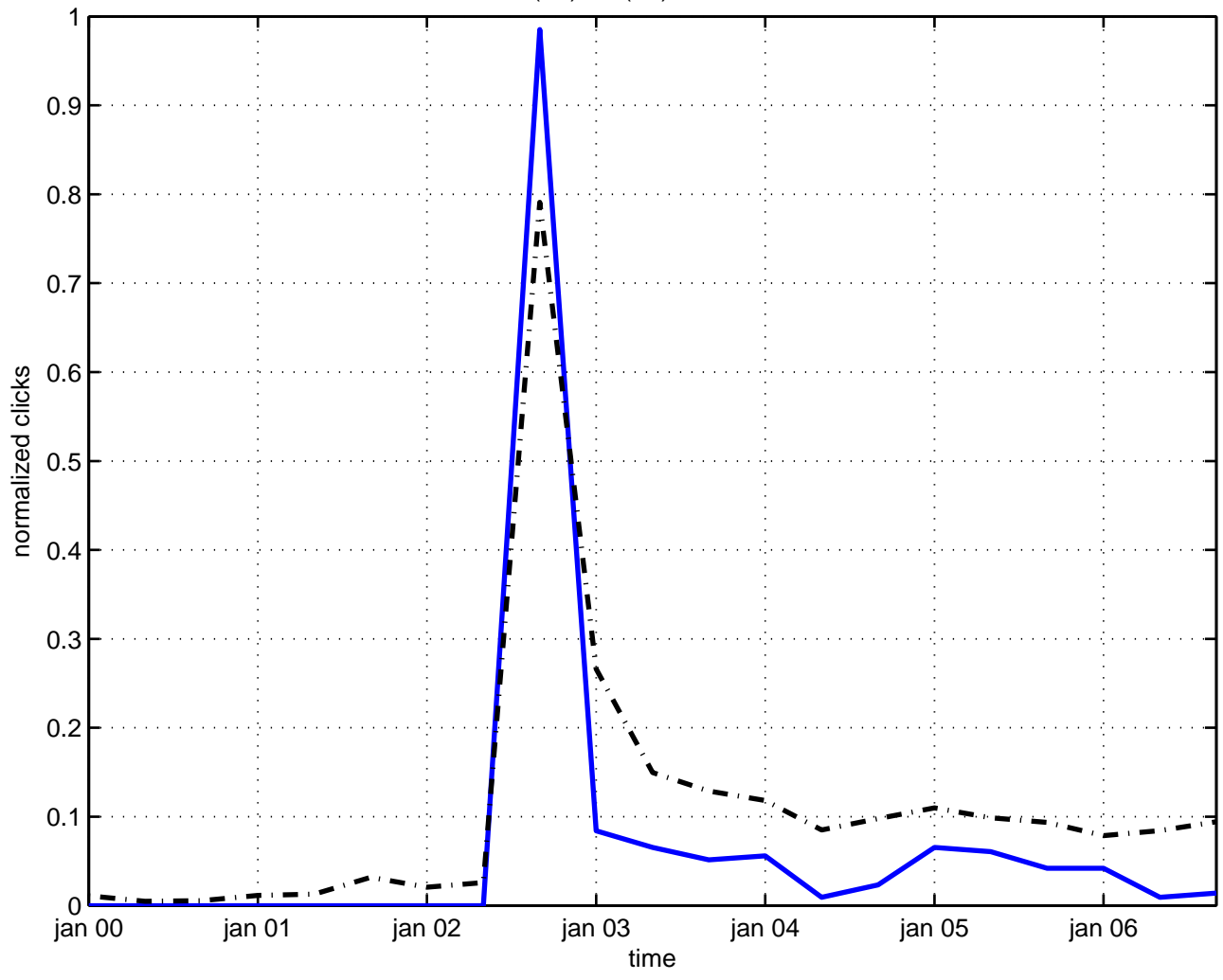
sl(2,r) x sl(2,r) invariance
