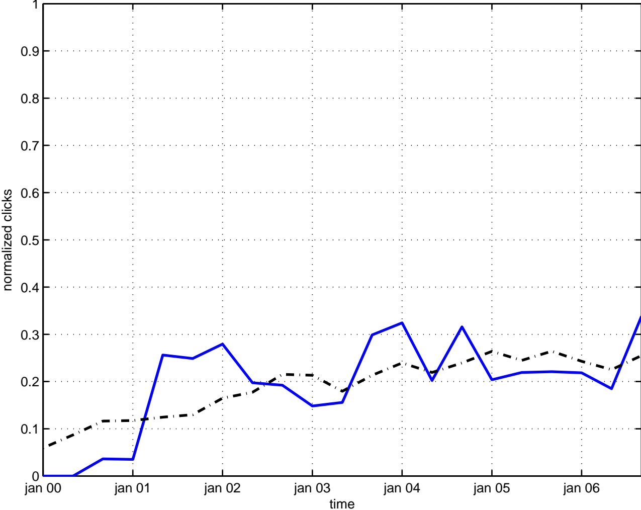
seiberg-witten map
