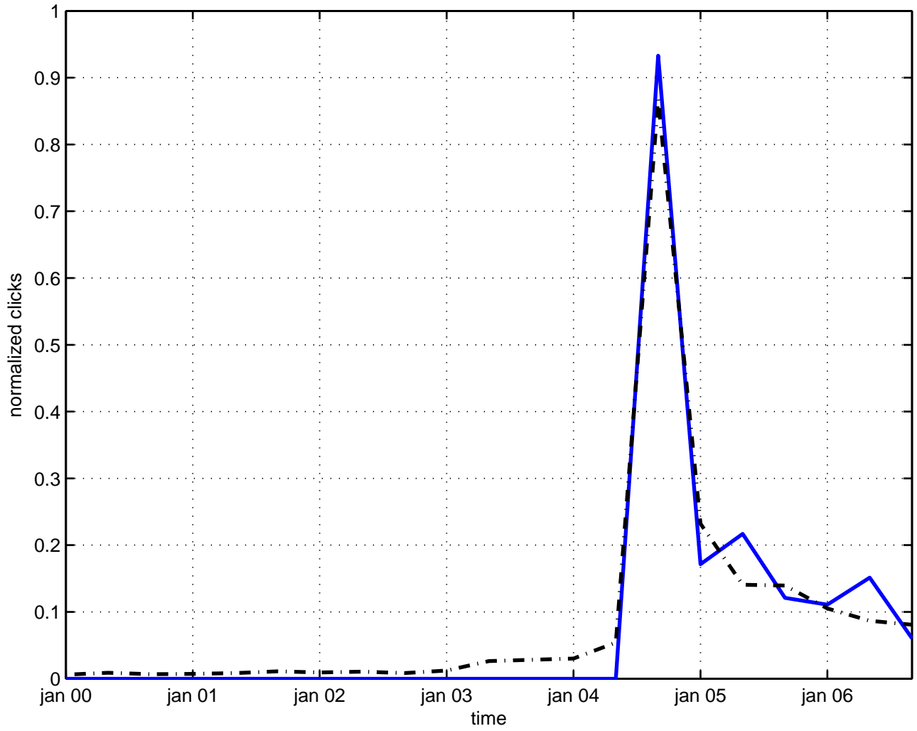
screening 't hooft loop
