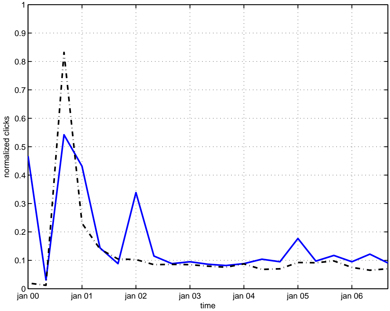
schwinger terms
