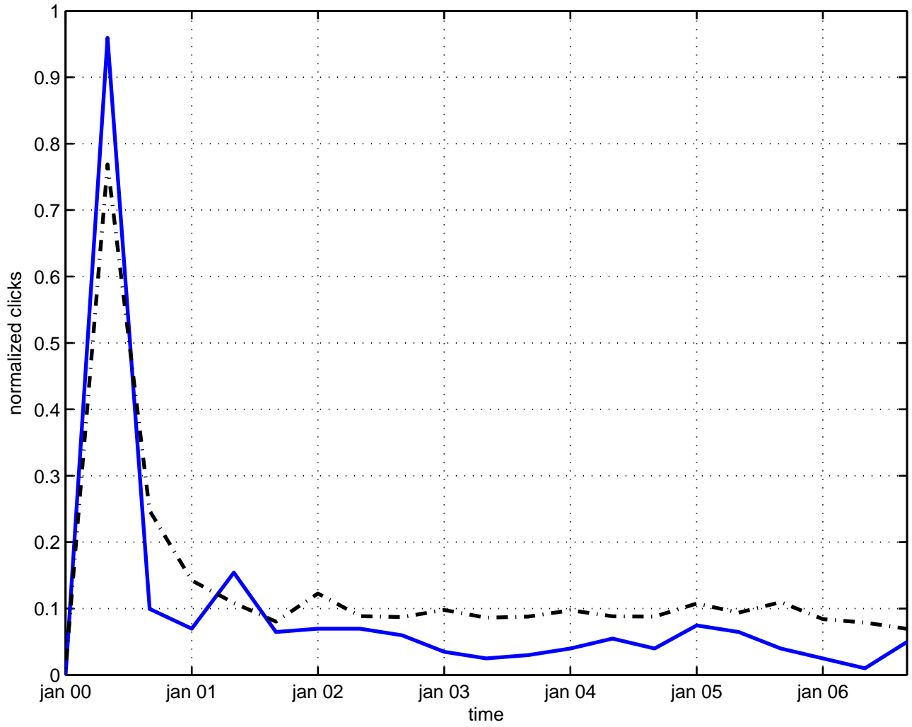
schwarzschild string
