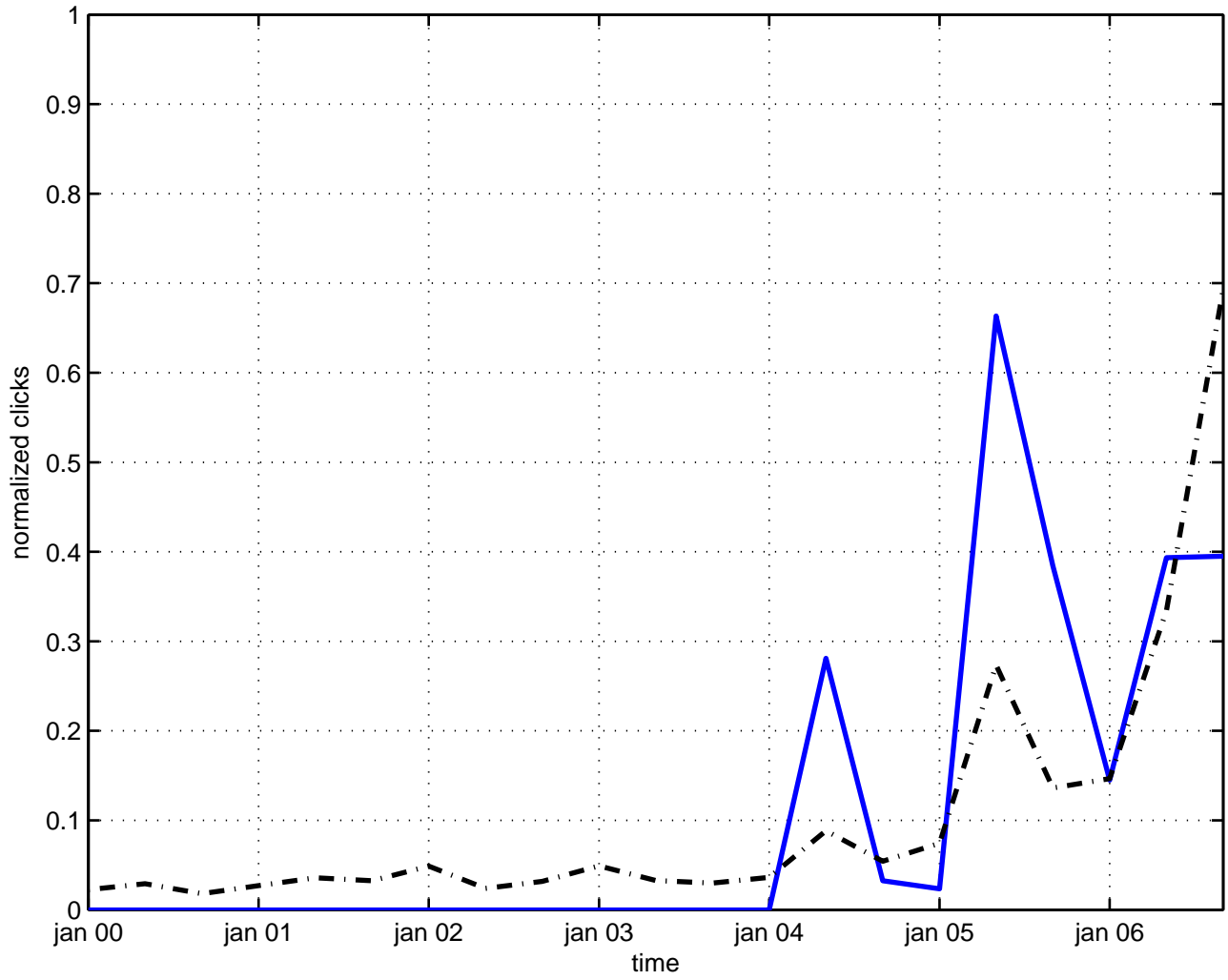
s-brane
