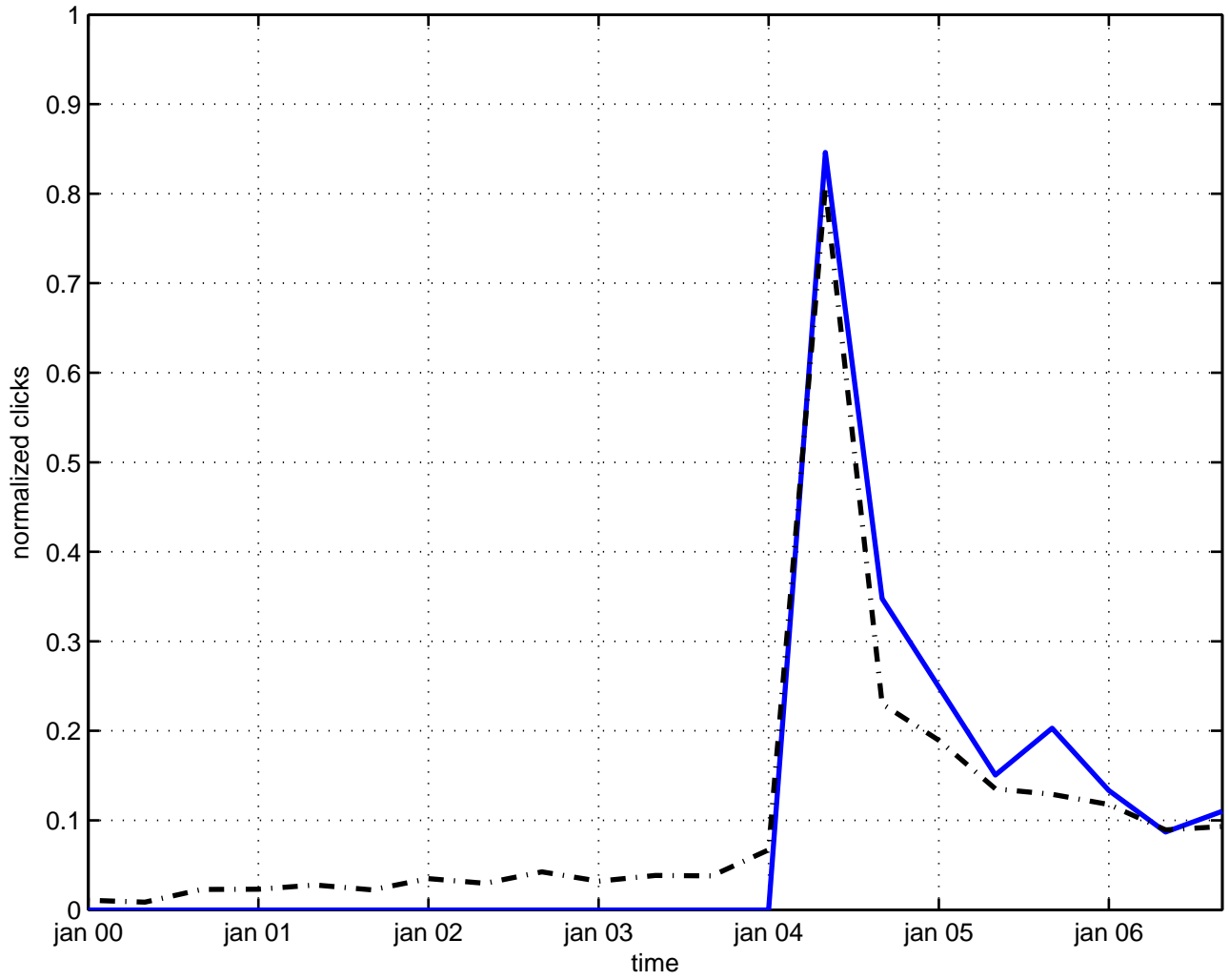
s(5)/z(n) space
