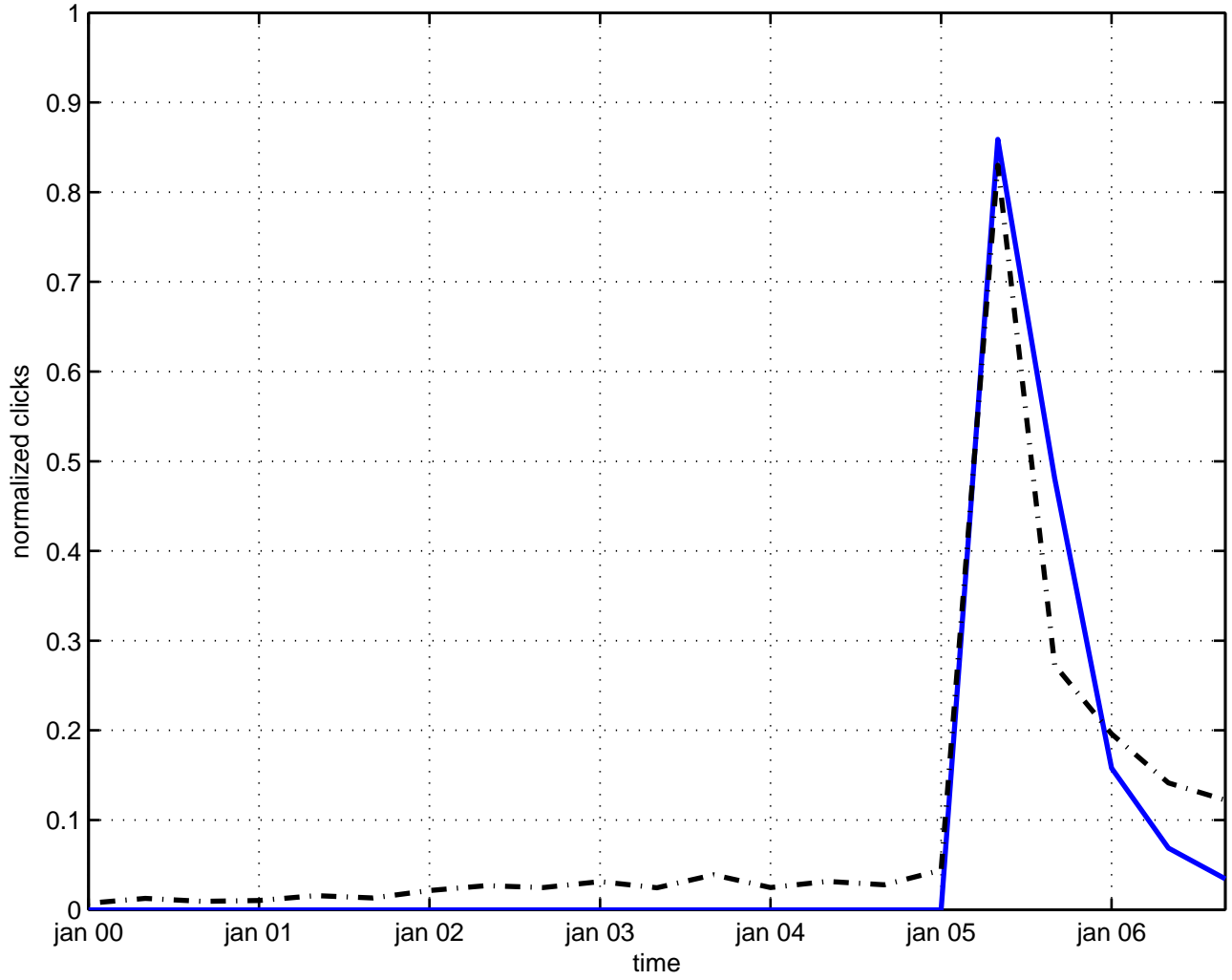
s(1)/z(2) compactification
