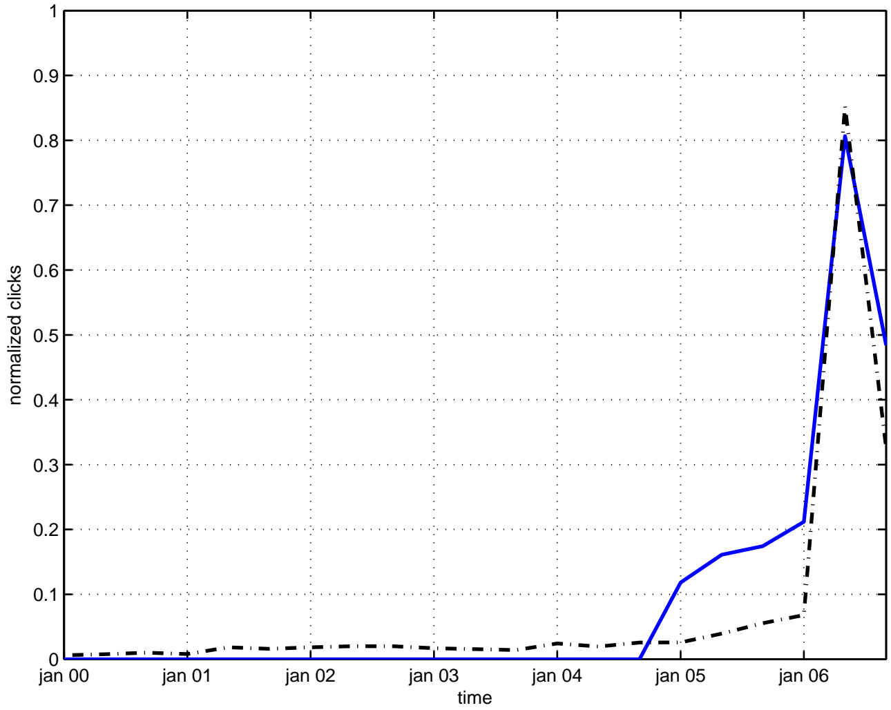
rotation black hole
