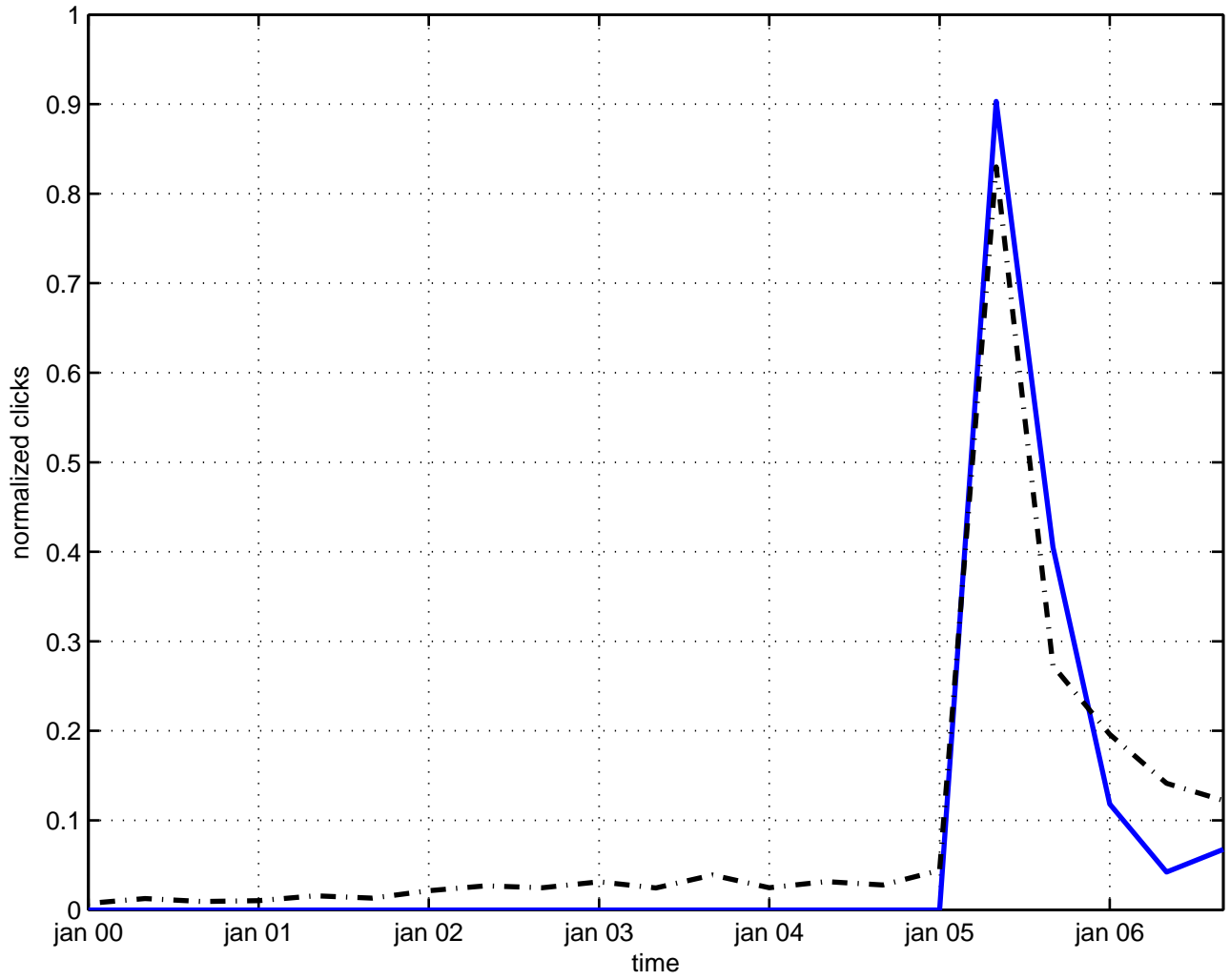
rho parameter
