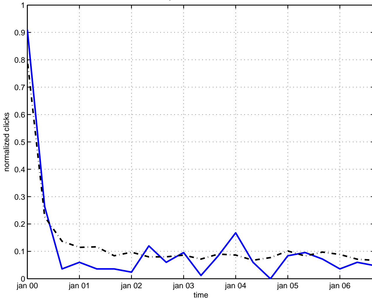
reparametrization time
