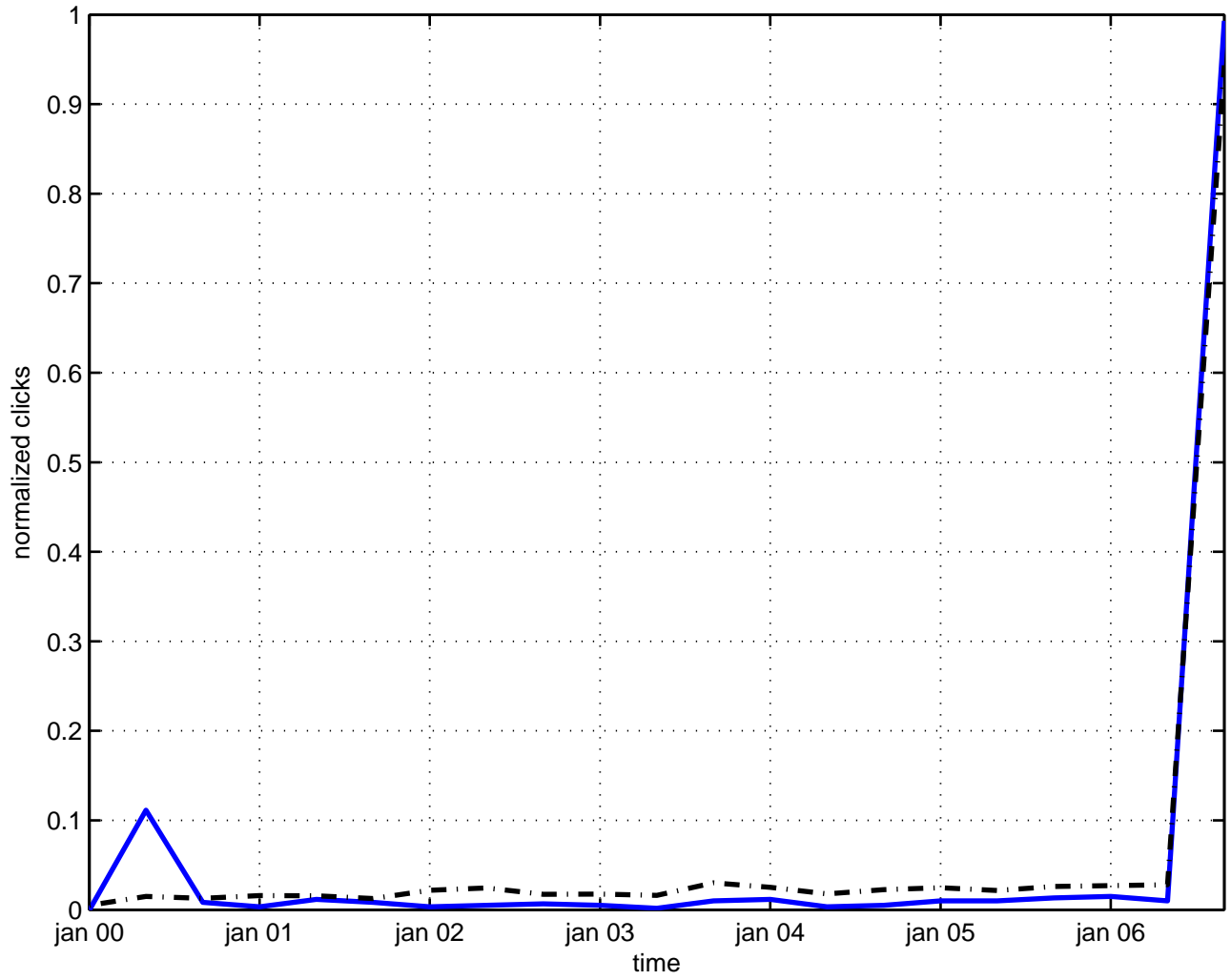
renormalizable quantum gravity
