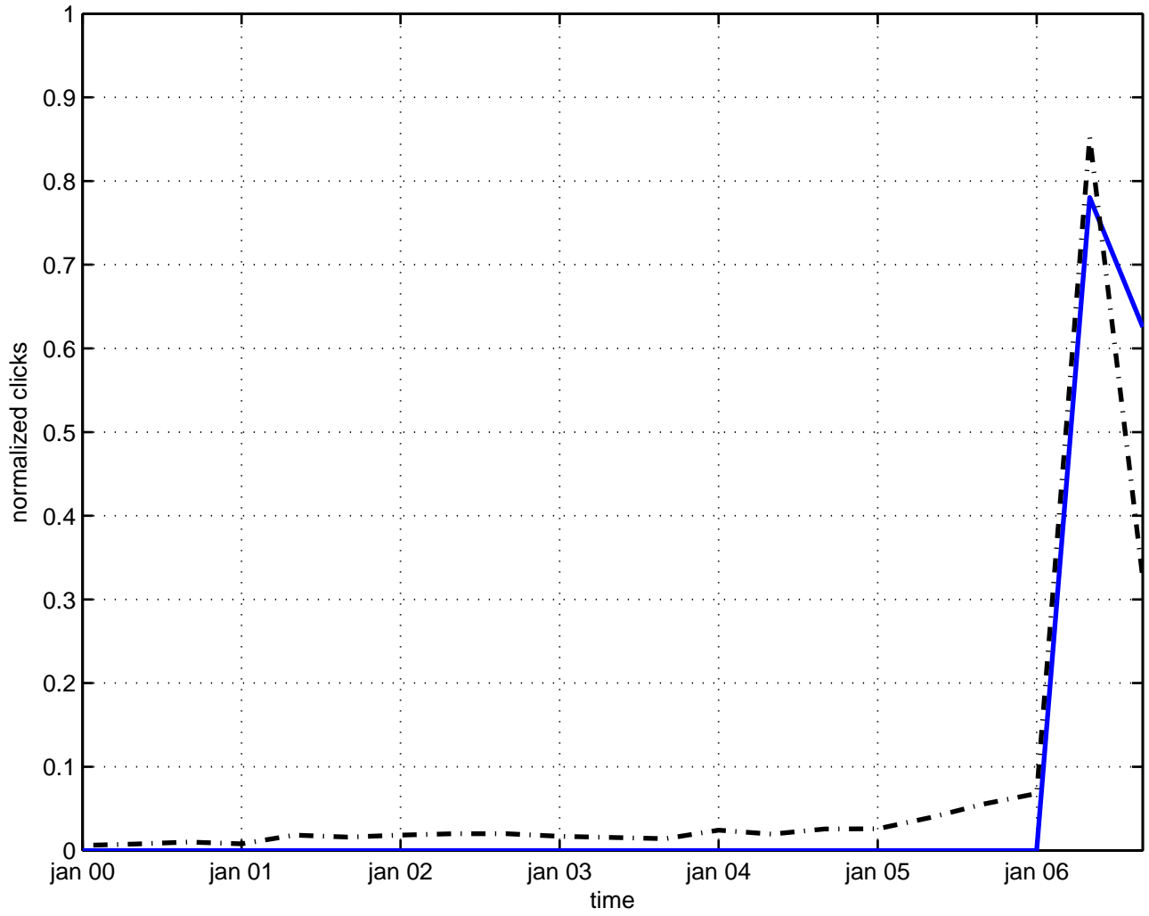
renormalizable gravitation
