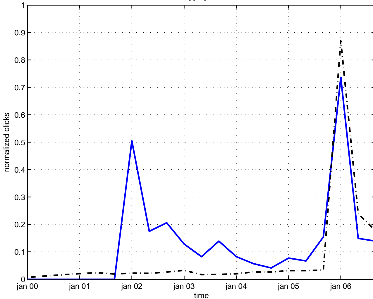
regge gluon
