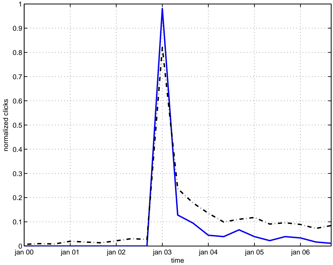
redshift supernova
