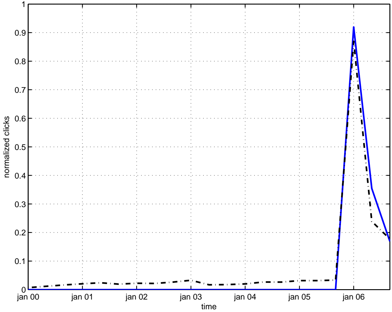
r(9) x t(2) space
