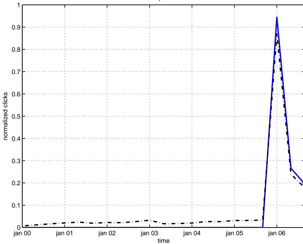
qubit
