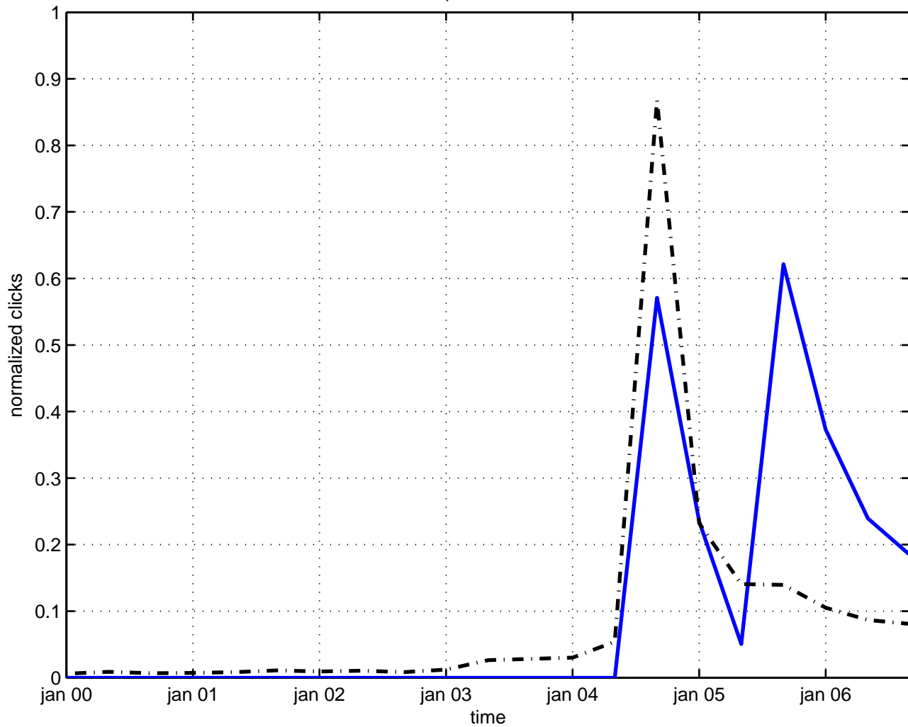
quarkonium
