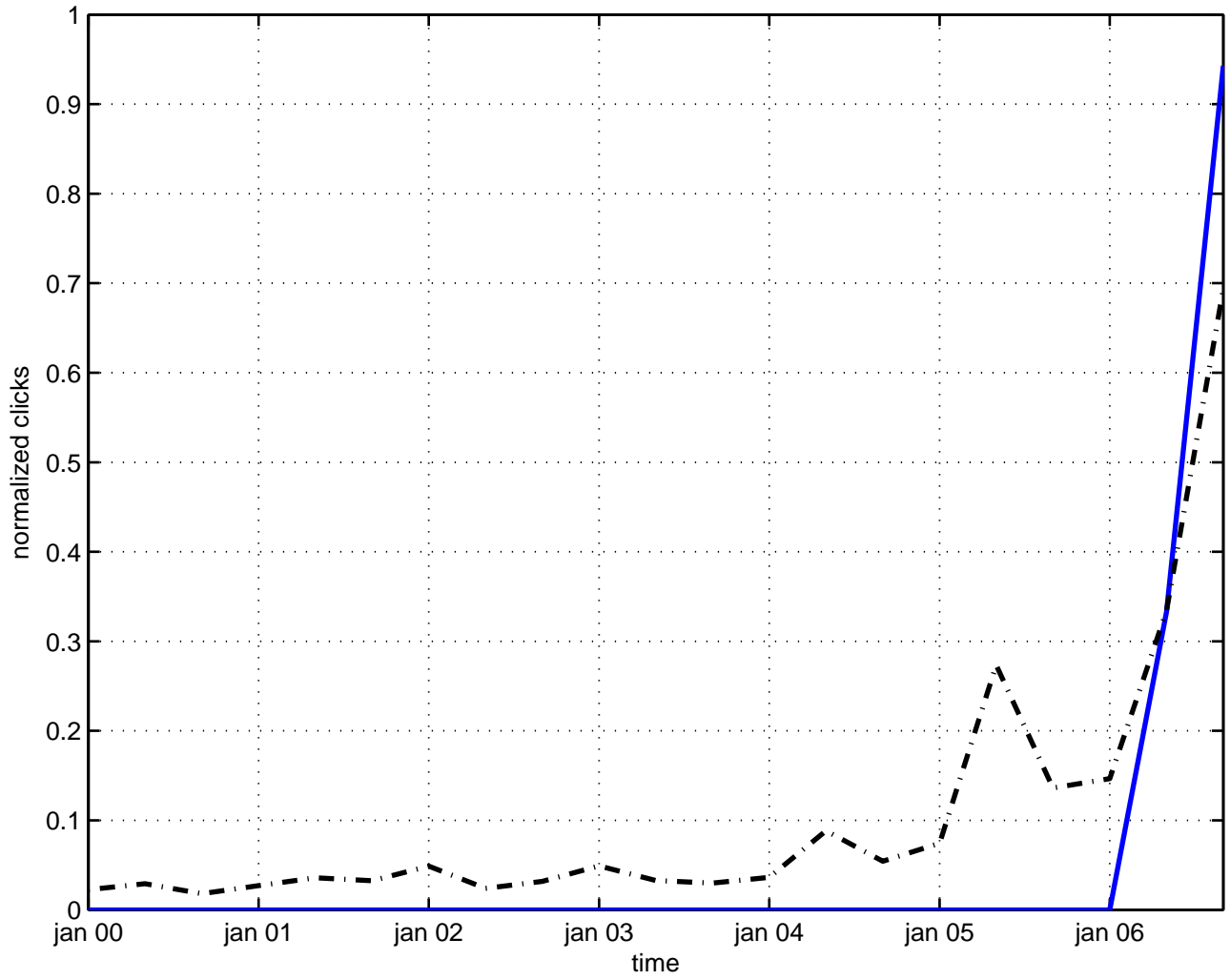
quark antiquark
