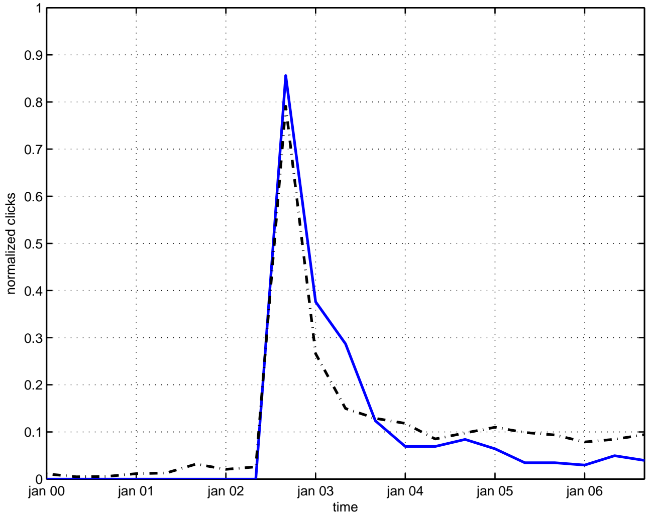
pseudoparticle
