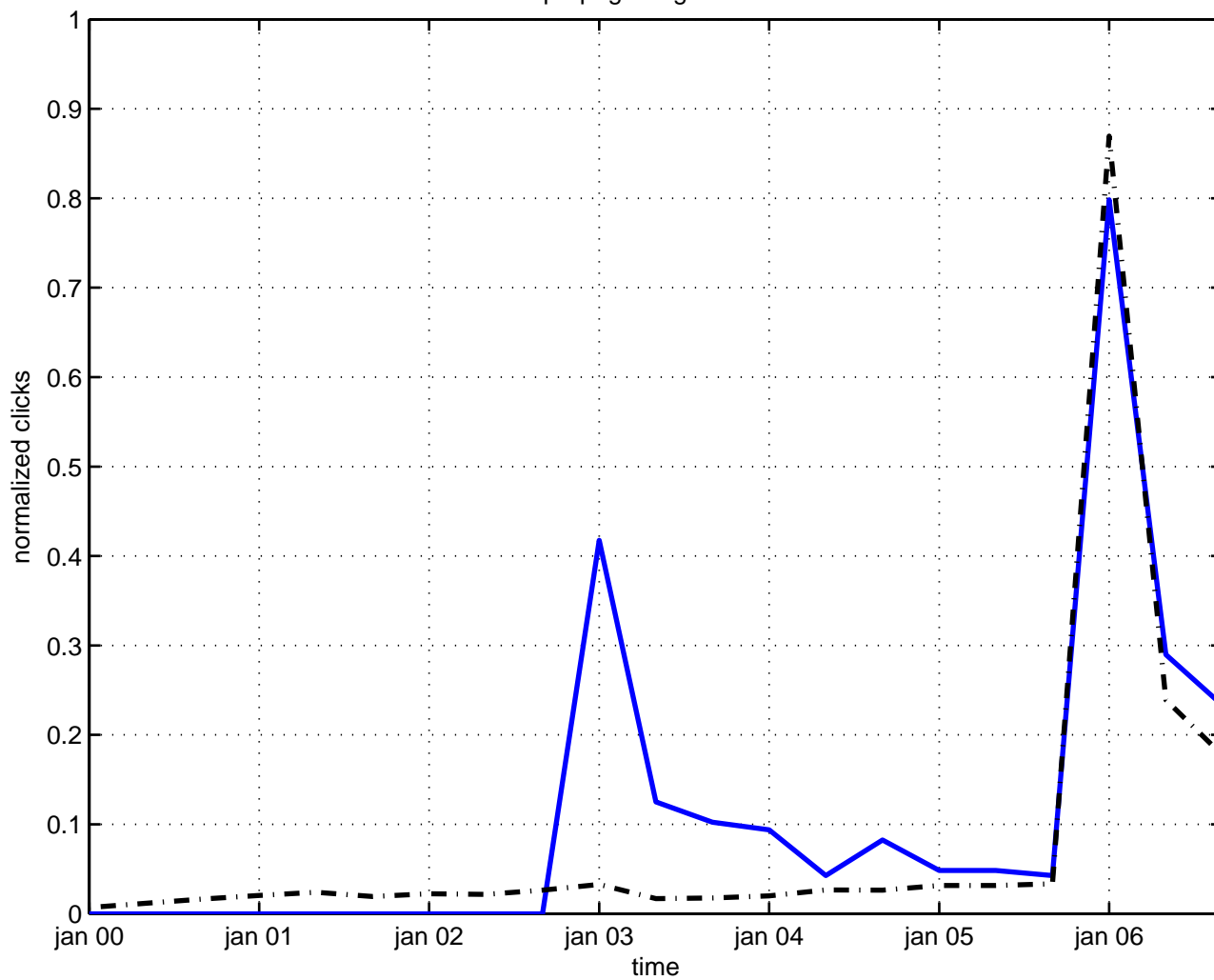
propagator gravitino
