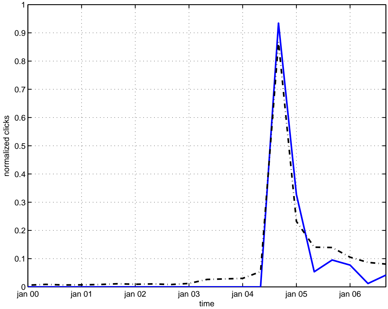
production soliton
