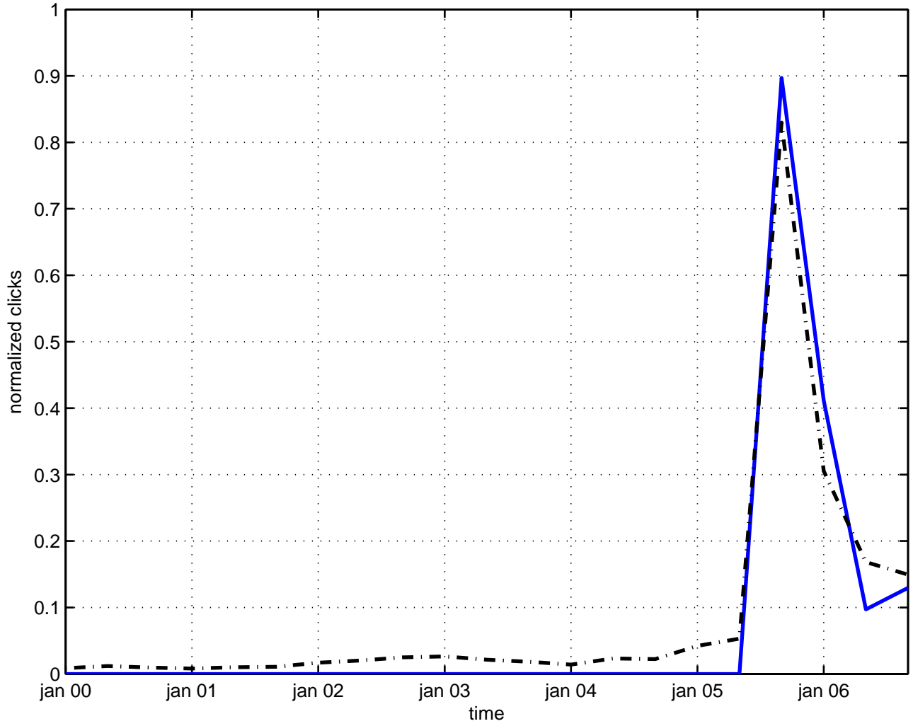
production fireball
