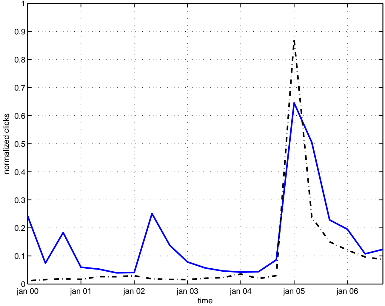
pomeron
