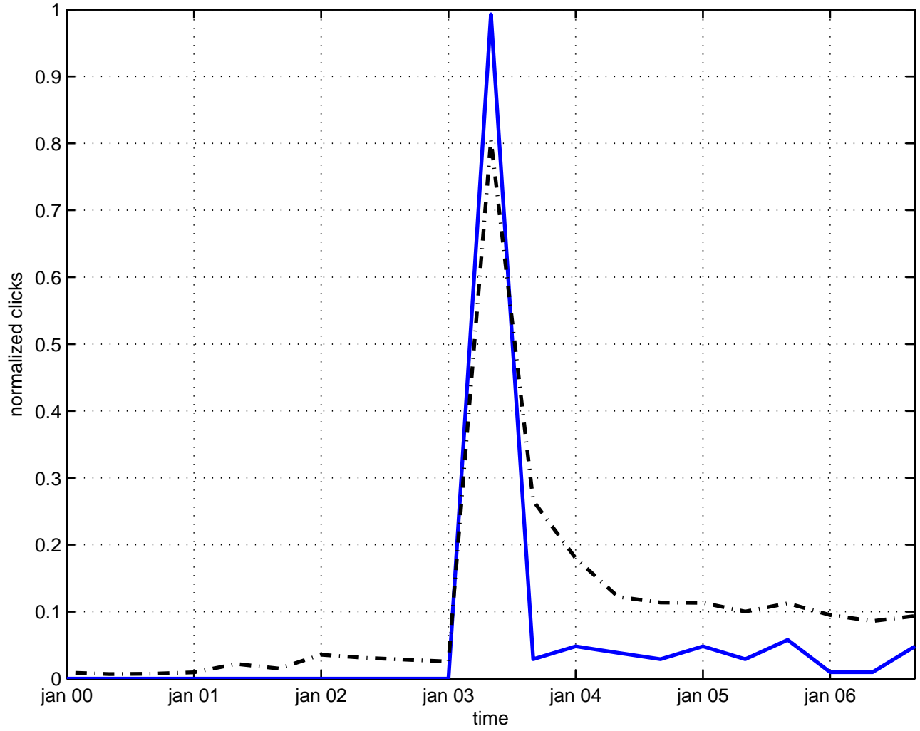
parity fermion
