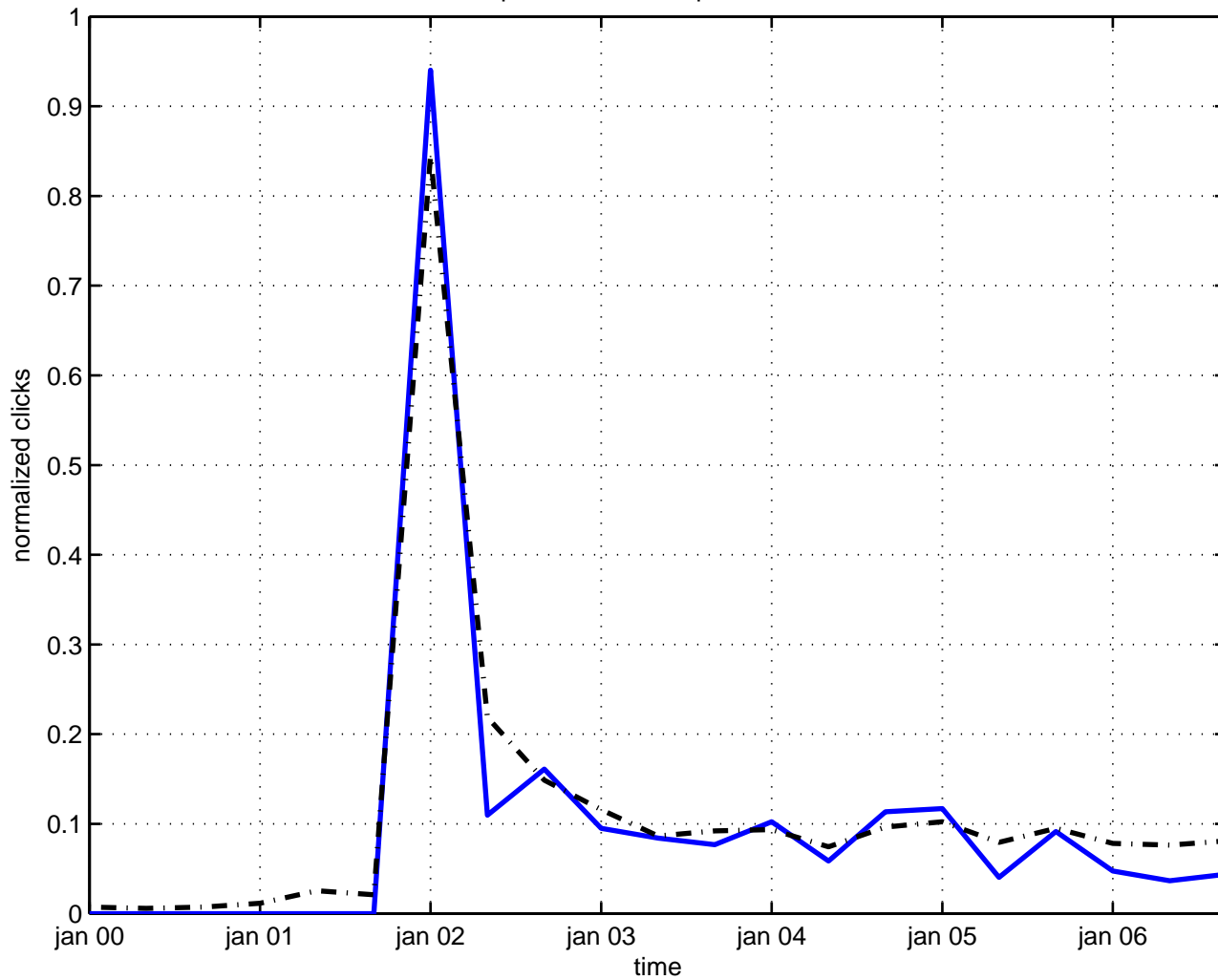
parametrization space-time
