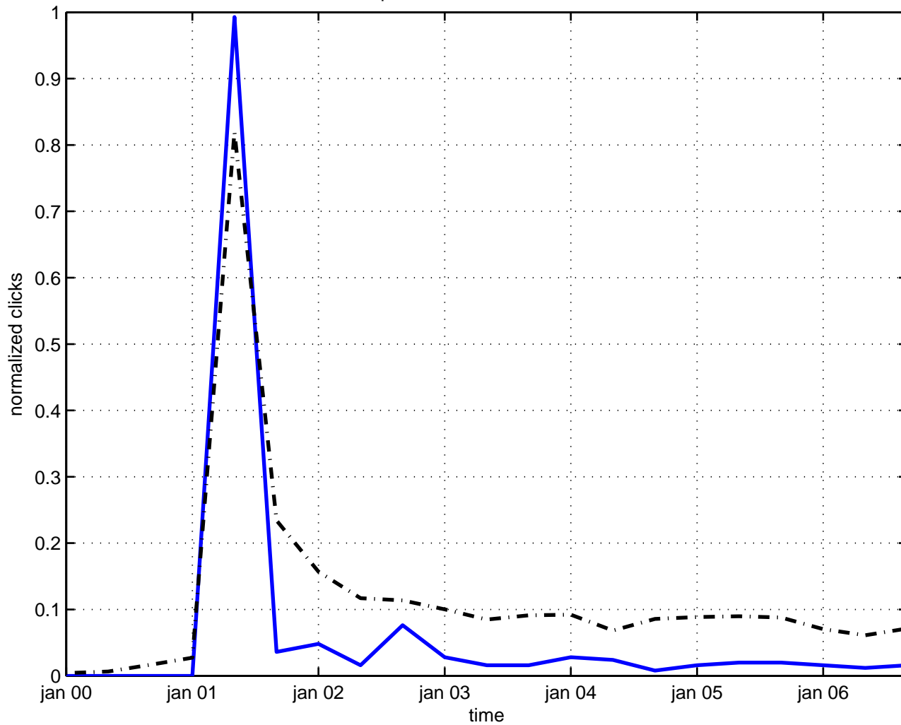
parametrization instanton
