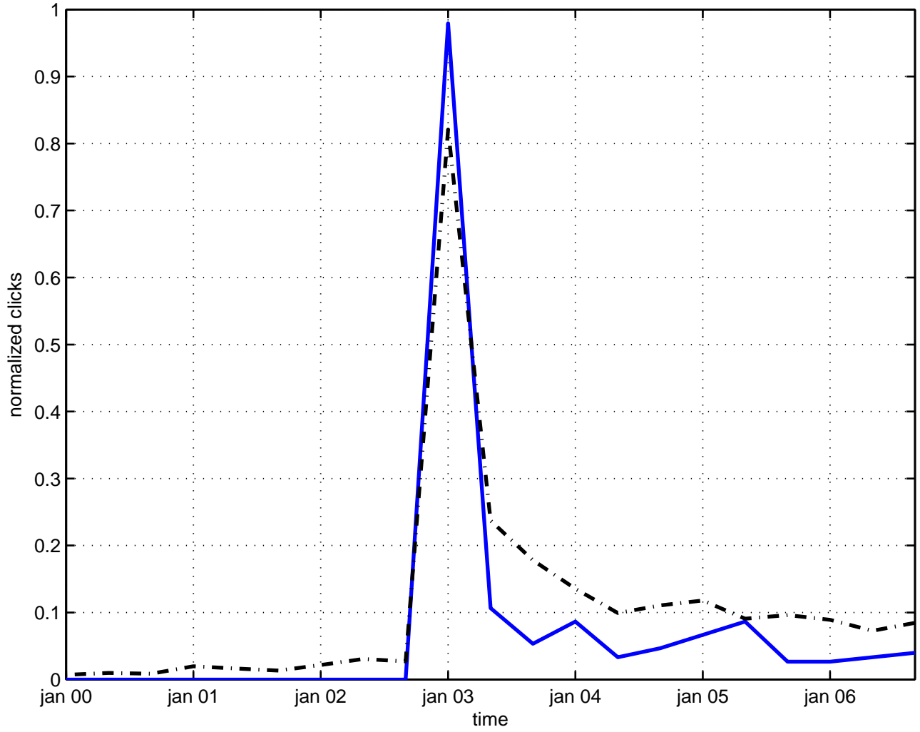
pair quark quark
