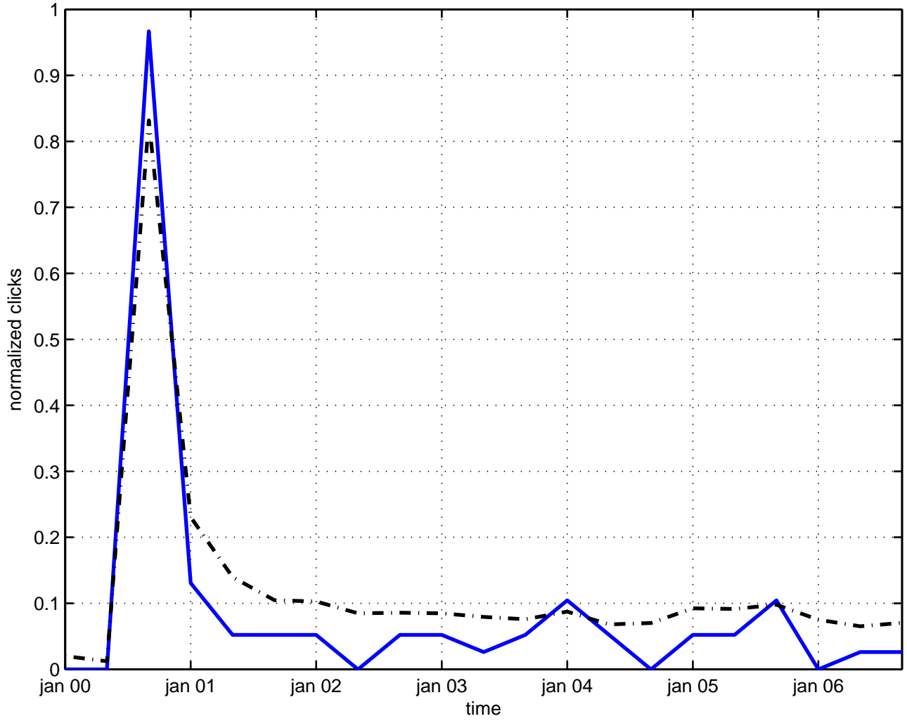
osp(1,2) invariance
